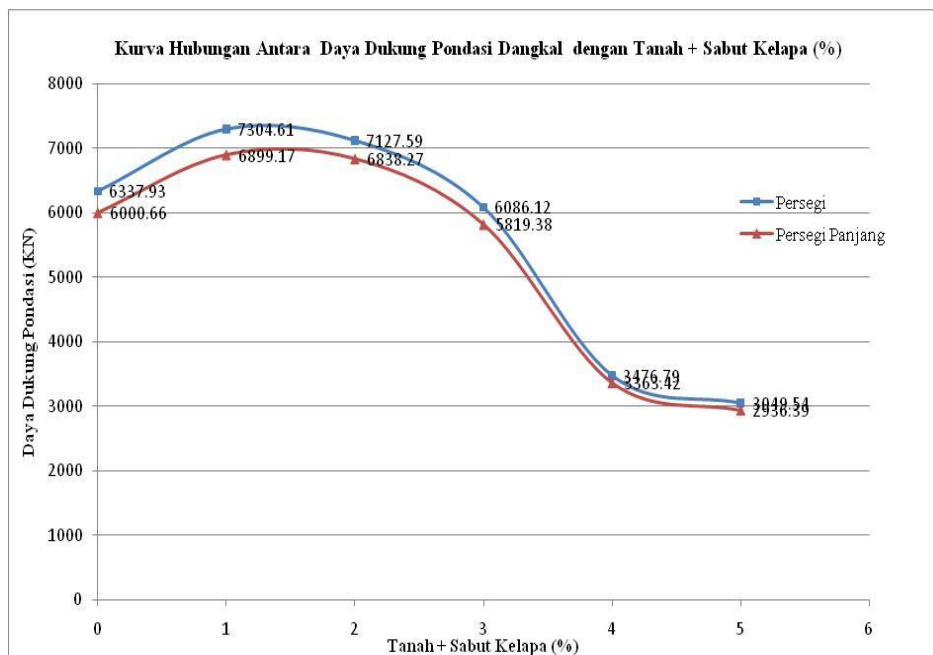
Gambar 2. Kurva Hubungan Daya Dukung Pondasi Dengan Tanah + Sabut Kelapa (0%-5%)
