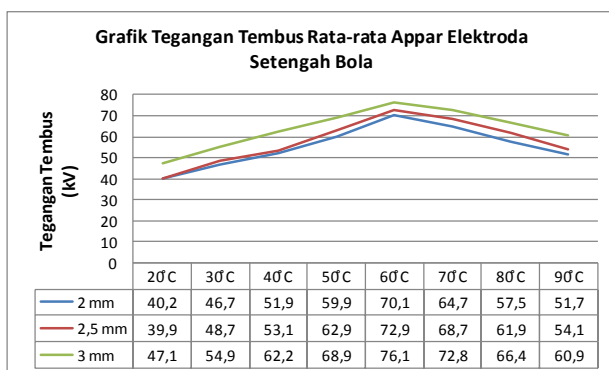
Gambar 4. Karakteristik tegangan tembus appar terhadap suhu
