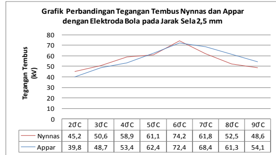
Gambar 13. Perbandingan karakteristik tegangan tembus nynnas dan appar dengan elektroda bola
