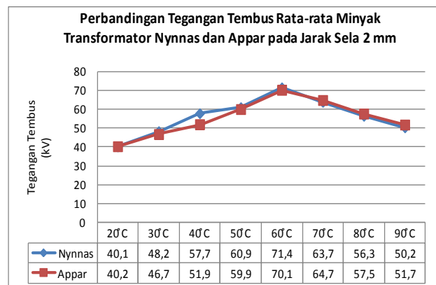
Gambar 6. Grafik perbandingan tegangan tembus minyak nynnas dan appar terhadap suhu minyak menggunakan elektroda setengah bola pada jarak 2 mm
