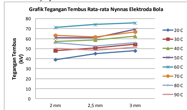
Gambar 10. Karakteristik tegangan tembus nynnas terhadap jarak sela
