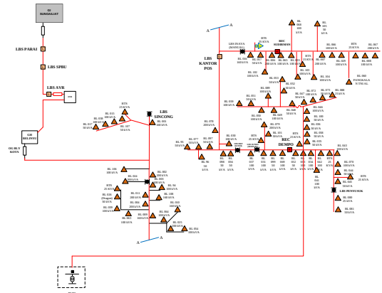
Gambar 4. Existing Single Line Diagram Penyulang dan Gardu Distribusi Belinyu (PT. PLN (Persero) Kantor Jaga Belinyu, 2016)
