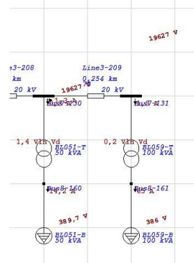
Gambar 8. Simulasi di Etap kondisi PLTD masuk sistem dan PLTS tidak masuk sistem.
