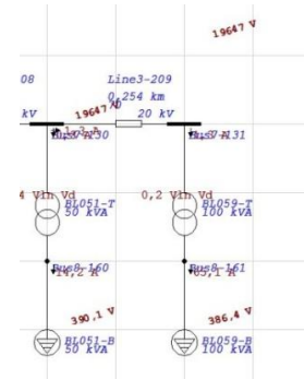
Gambar 7. Simulasi di Etap 12.6 kondisi PLTD dan PLTS masuk sistem
