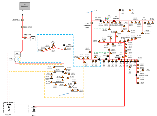
Gambar 5. Rencana Feeder baru dan PLTD (PT. PLN (Persero) Kantor Jaga Belinyu, 2017)
