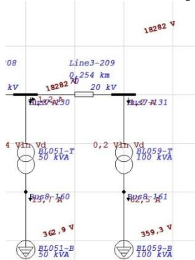
Gambar 9. Simulasi di Etap kondisi PLTD keluar sistem dan PLTS masuk sistem.
