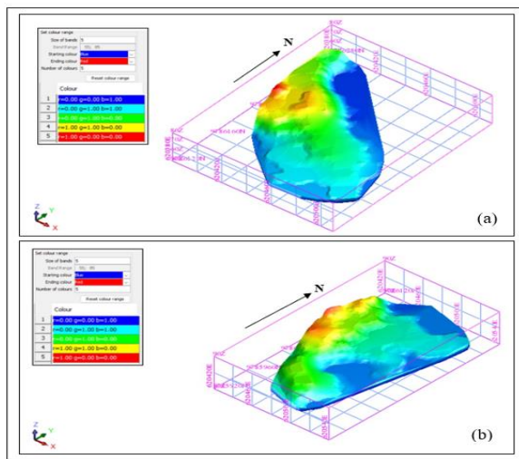
Gambar 6. Bentuk Digital Terrain Model DTM Surface : (a) Blok A, (b) Blok B
