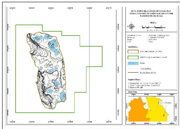
Gambar 3. Peta topografi menggunakan pengukuran terestris
