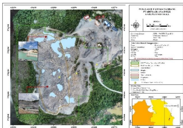
Gambar 2. Peta situasi wilayah IUP menggunakan drone
