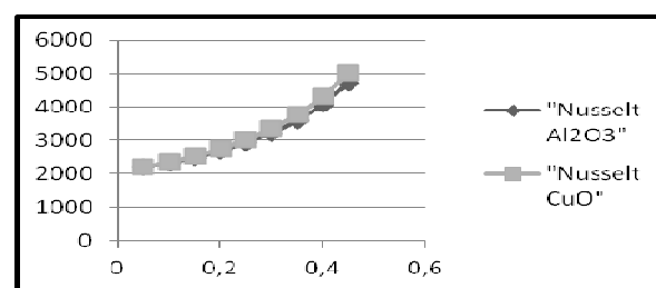
Gambar 3. Grafik Hubungan Fraksi Volume dengan Bilangan Nusselt
