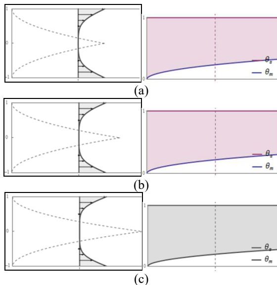
Gambar 4. Pola aliran dan temperatur \text{Al}_2\text{O}_3 dengan fraksi volume: (a) 10%, (b) 20%, dan (c) 30%.
