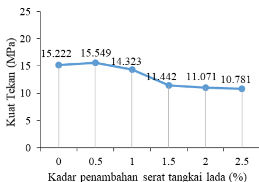
Gambar 2. Kuat tekan beton serat tangkai lada pada usia beton 7 hari
