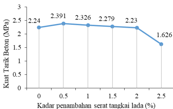
Gambar 4. Kuat tarik belah beton serat tangkai lada pada usia beton 28 hari
