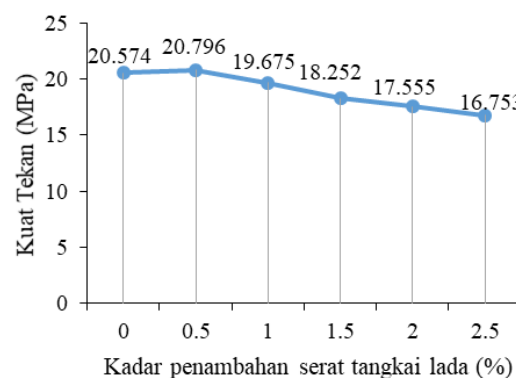
Gambar 3. Kuat tekan beton serat tangkai lada pada usia beton 28 hari
