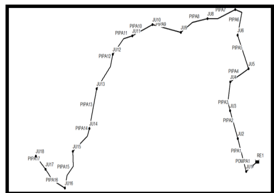
Gambar 2. Jaringan Pipa Transmisi
