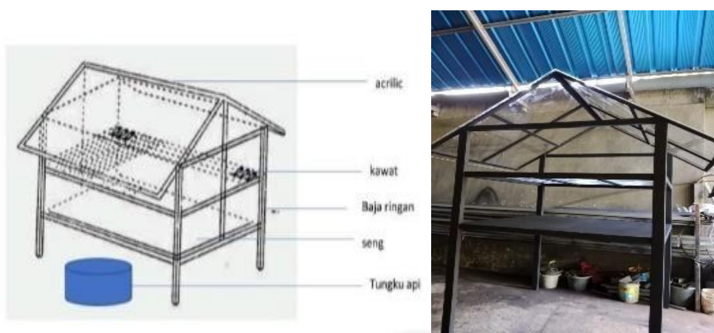
Gambar 2, Desain alat pengering hybrid dan alat pengeringan hybrid (Bidayani, et al , 2022)
